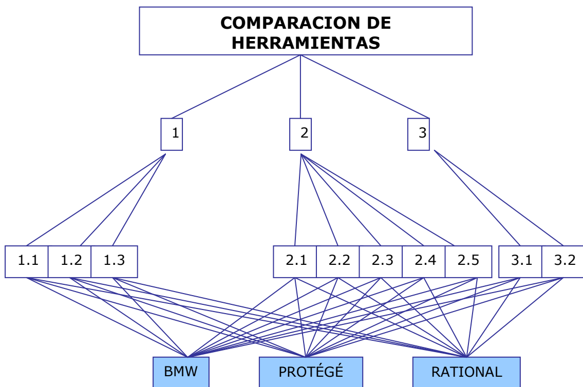
Figura 6.3. Modelo jerárquico AHP – comparación herramientas
