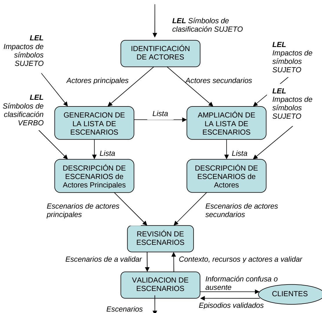
Figura 3.5. Etapas para la construcción de escenarios a partir del LEL [Hada 1997]
