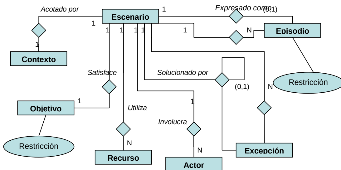
Figura 3.3. Diagrama de entidad-relación para el modelo de escenarios [Leite 1997]
