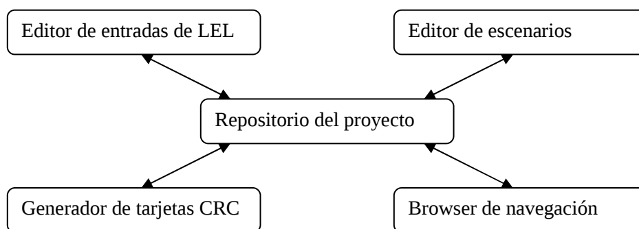
Figura 3.6. Arquitectura de Baseline Mentor Workbench [Antonelli 2003]
