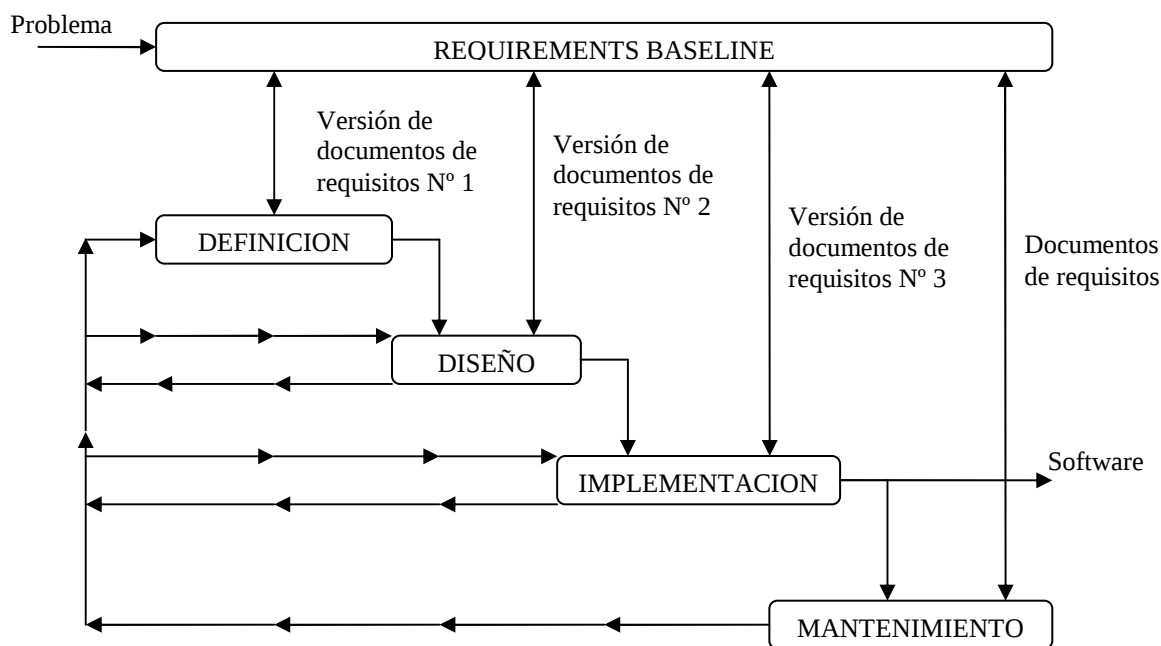
Figura 3.1. Requirements baseline y el proceso de desarrollo de software [Leite 1995]
