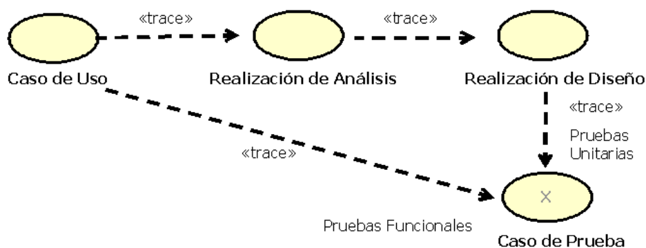
Figura 5.2. Trazabilidad a partir de los Casos de Uso
