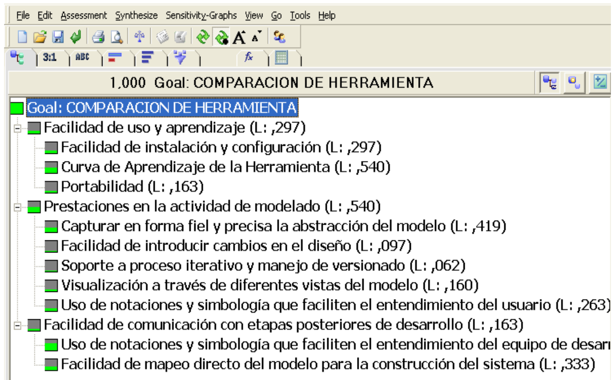
Pantalla 7.10. Expert Choice - comparación de herramientas para AHP
