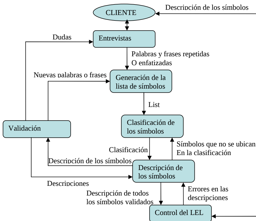
Figura 3.4. Etapas para la construcción del LEL [Hada 1997]
