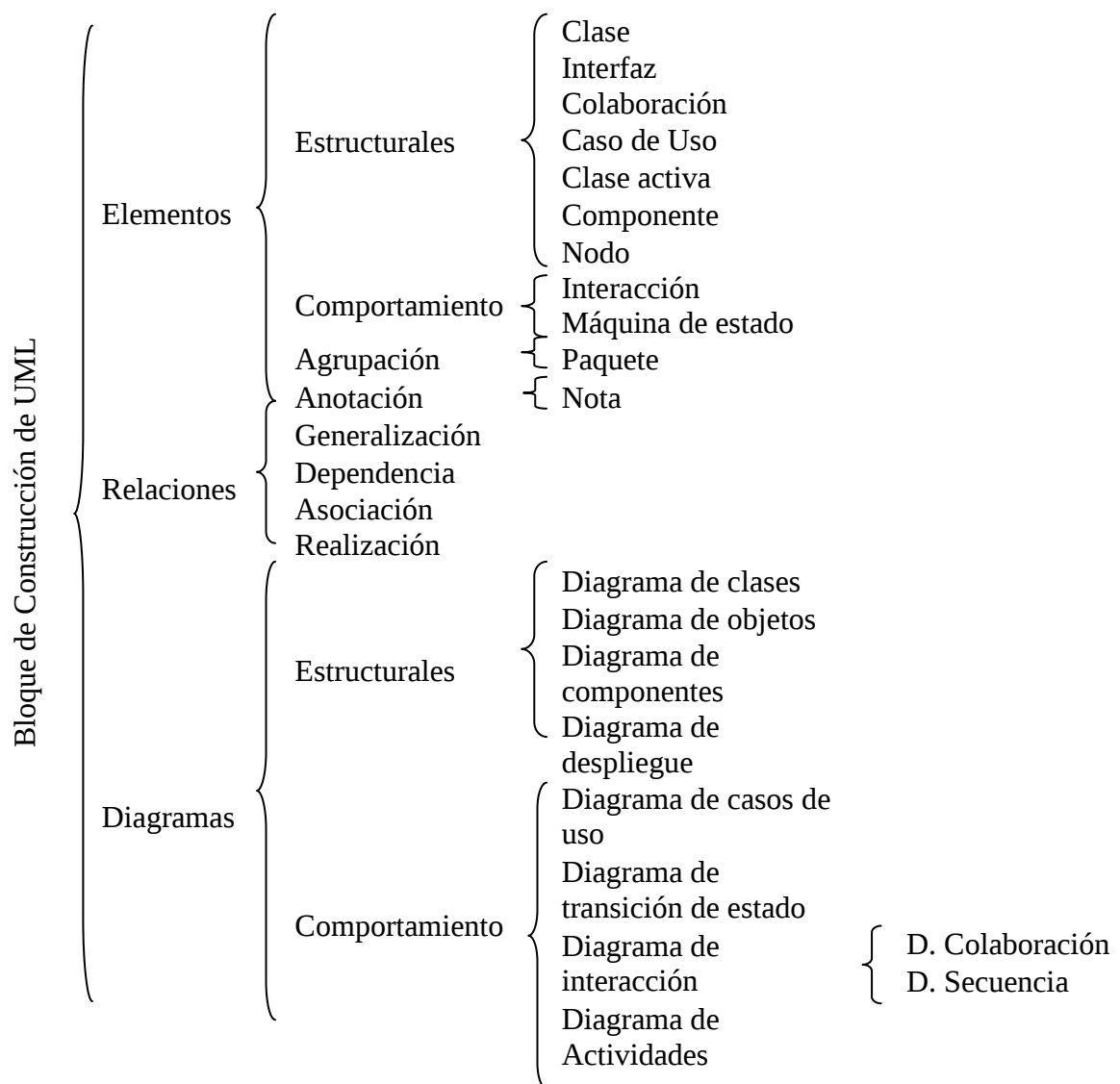
Figura 5.7. Bloques de Construcción de UML
