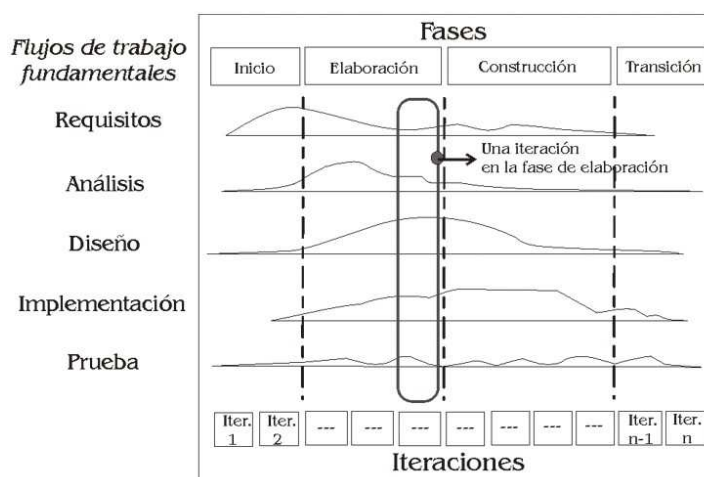
Figura 5.5. Esfuerzo en actividades según fase del proyecto
